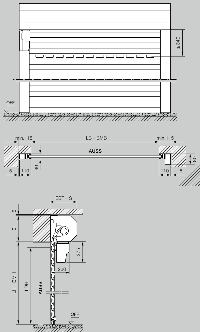
Belső és külső szerelésű redőnykapuk mérettartománya
